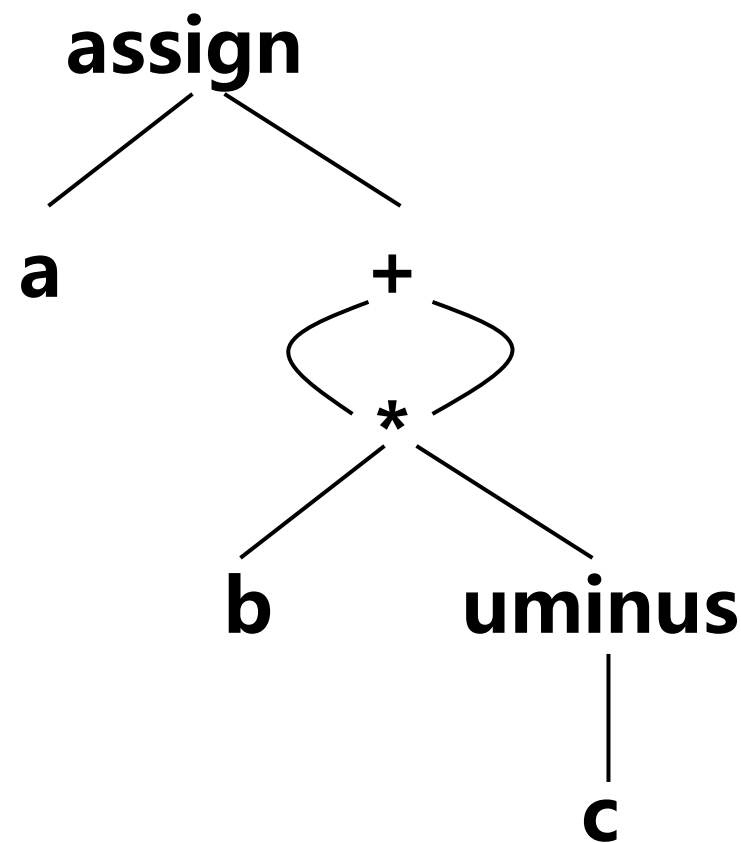
DAG
